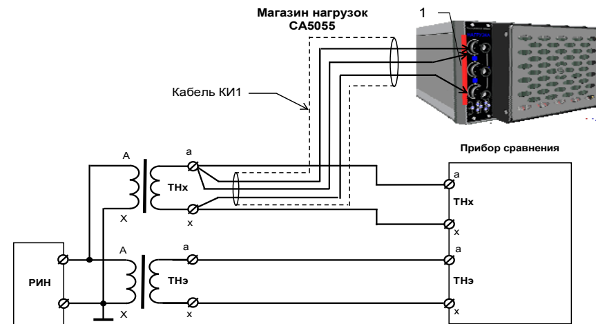
1 – клеммы Магазина для подключения ТН (X1, X2, X3 – сверху вниз); РИН – регулируемый источник трехфазной системы напряжений; ТНх – поверяемый или калибруемый трансформатор напряжения; ТНэ – эталонный трансформатор напряжения
