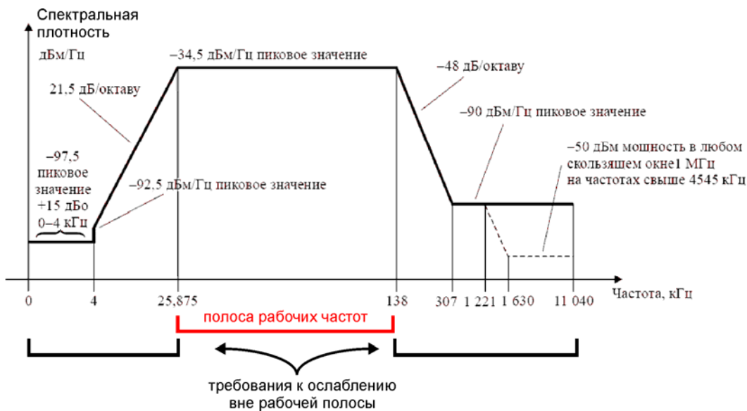
Рис. 31. Спектральная маска передатчика абонента ADSL и ADSL2.
