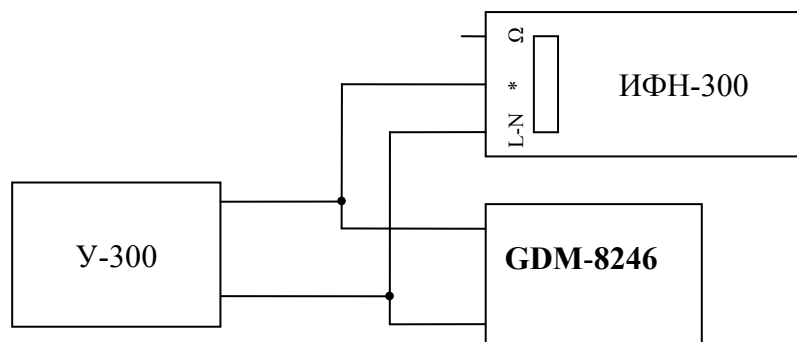
Рисунок 6.7.1 – Схема проверки погрешности при измерении напряжения
