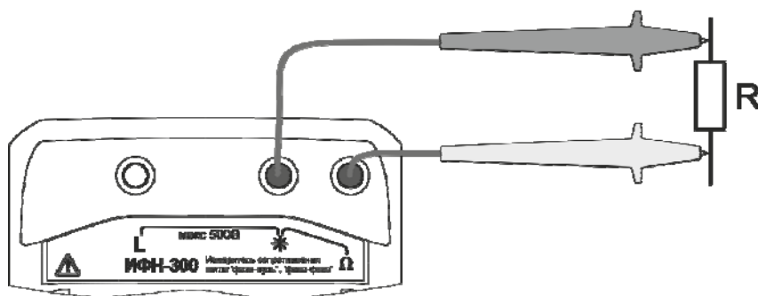
Рисунок 2.4.3.1 - Измерение сопротивления металlosвязи
