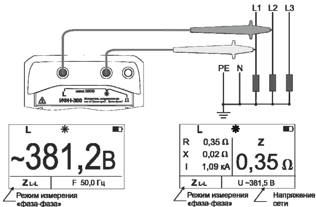
Рисунок 2.4.2.2 Схема подключения и вид индикатора при измерении сопротивления петли «фаза-фаза»
