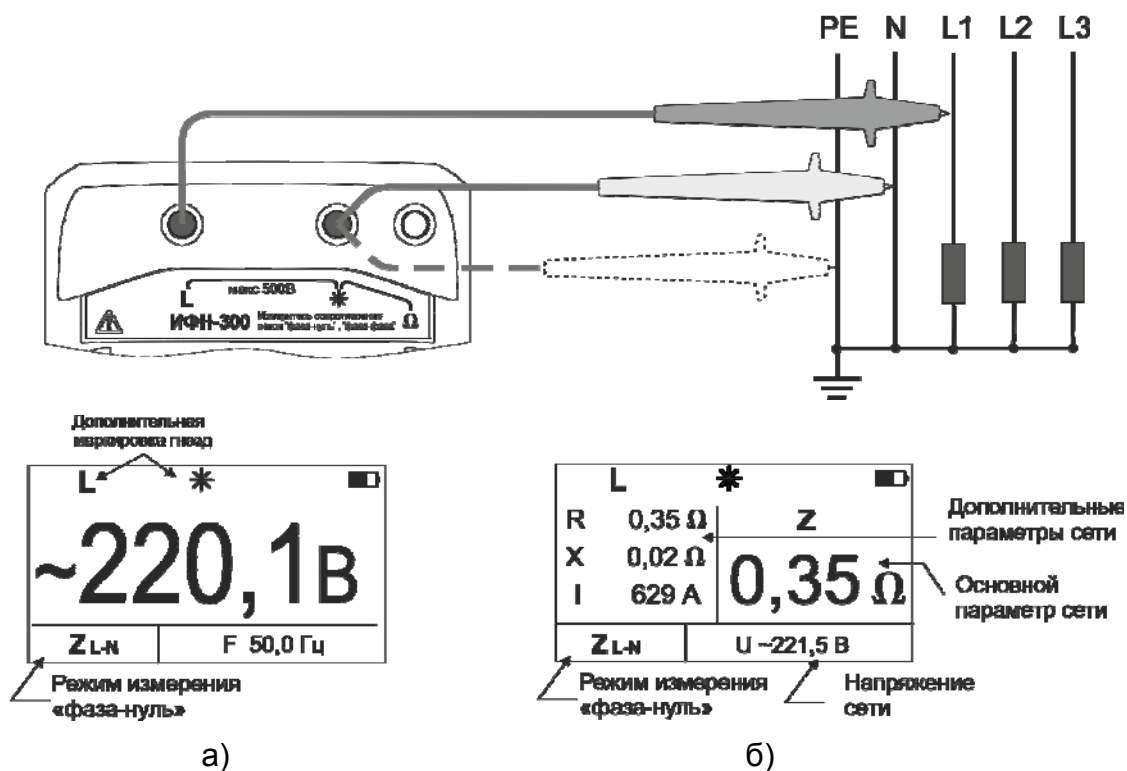
Рисунок 2.4.2.1 Схема подключения и вид индикатора при измерении сопротивления петли «фаза-нуль»
