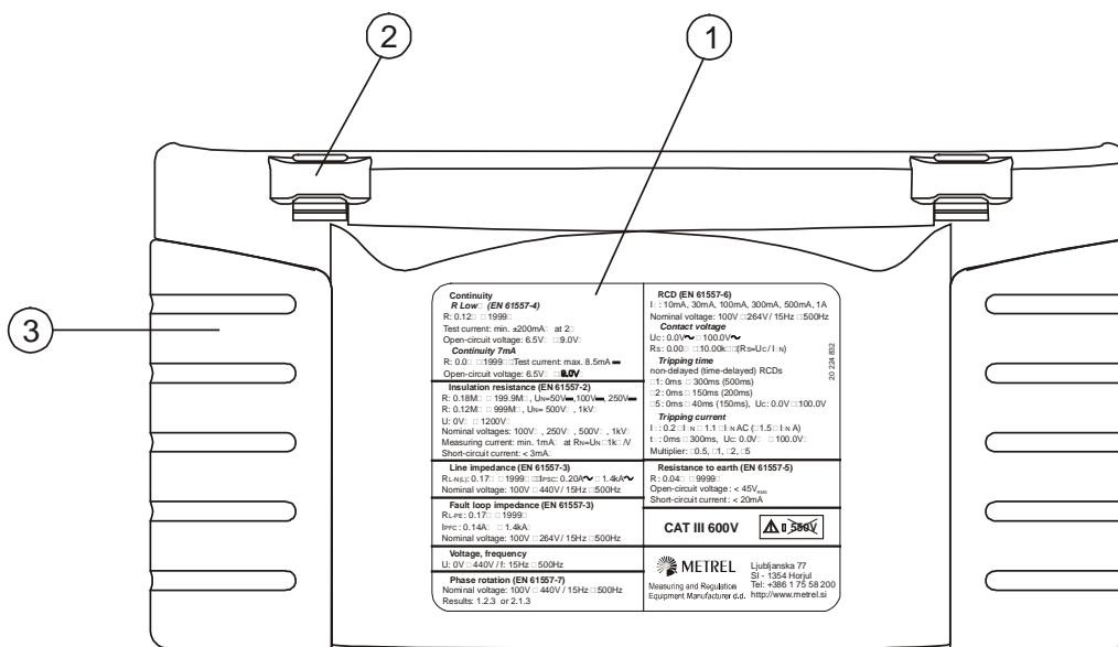
Рисунок 3.5: Низ
