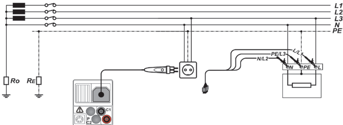
Рисунок 5.54: Подключение штепсельного щупа «plug commander» и 3-х проводного тестового кабеля
