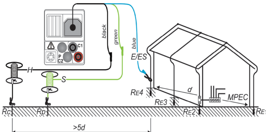
Рисунок 5.37: Сопротивление заземления, измерение сопротивления системы молниезащиты
