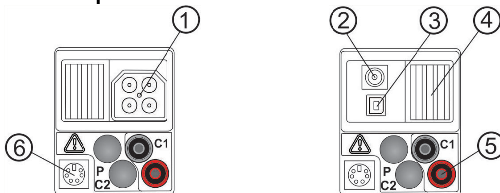
Рисунок 3.2: Панель разъемов
