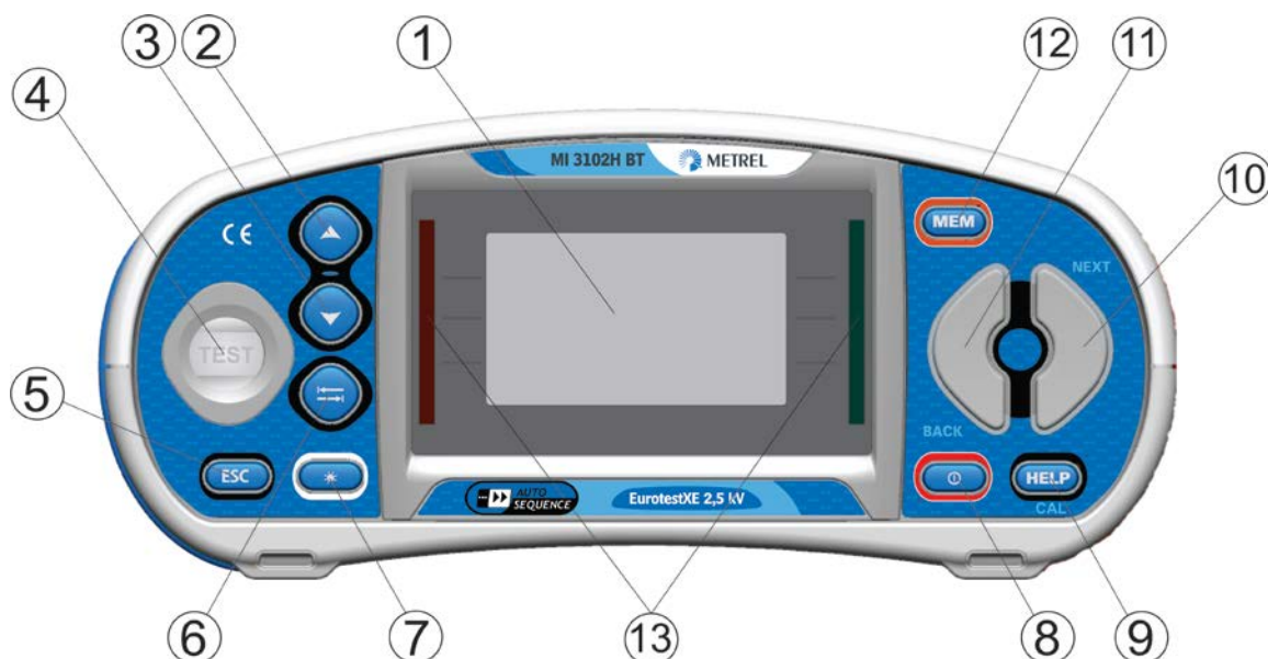
Рисунок 3.1: Передняя панель
