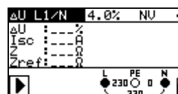
Рисунок 5.30: Падение напряжения
