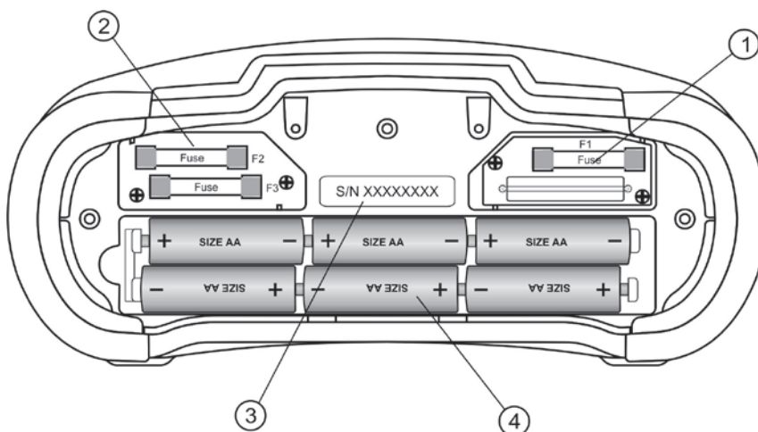
Рисунок 3.4: Батарейный отсек и отсек с плавкими предохранителями
