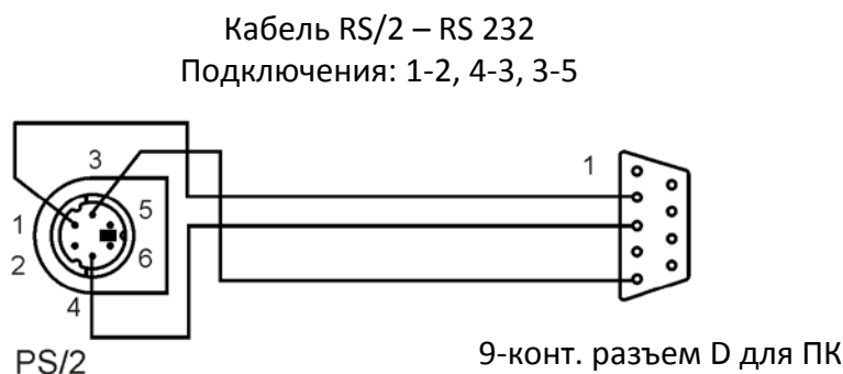
Рисунок 7.14: Подключение для передачи данных через COM – порт ПК
