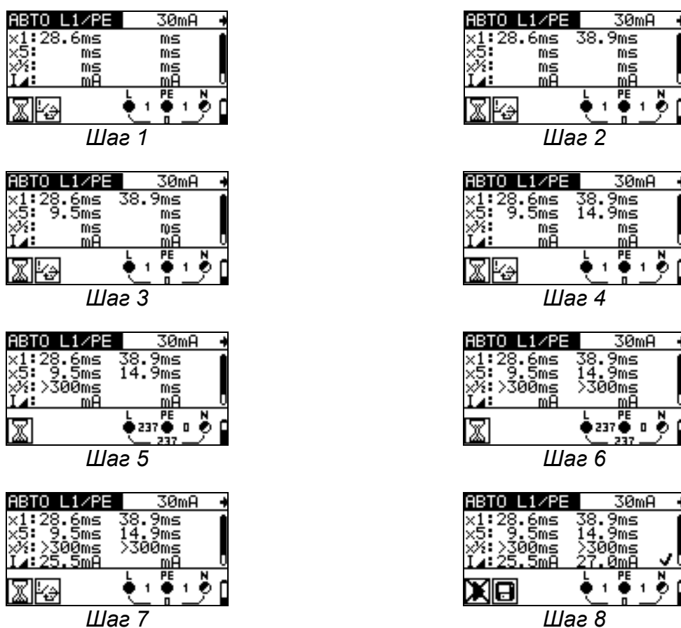
Рисунок 5.24: Отдельные шаги автоматических испытаний УЗО
