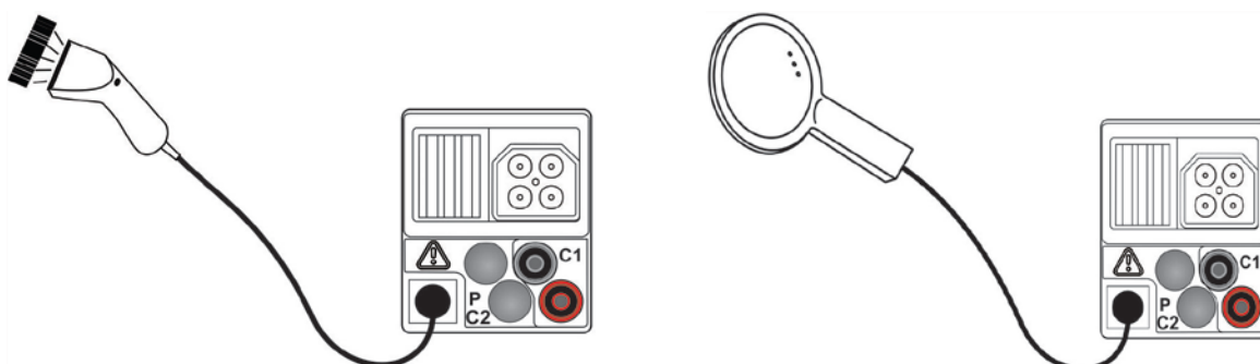
Рисунок 7.13: Подключение считывателя штрих-кодов и считывателя радиометок RFID
