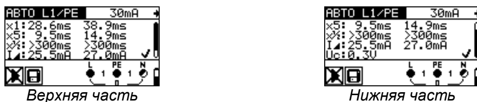
Рисунок 5.25: Две части поля с результатами при автоматической проверке УЗО
