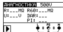
Рисунок 5.9: Меню диагностических испытаний
