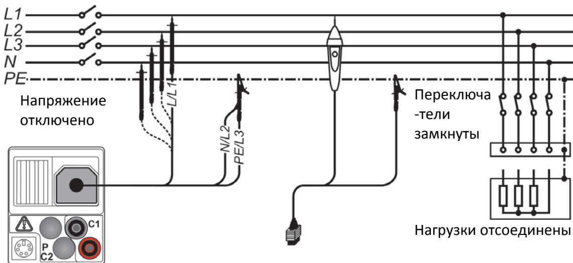
Рисунок 5.6: Подключение 3-х проводного тестового кабеля и щупа с наконечником «Тир commander» ( U_N \leq 1 \text{ кВ} )
