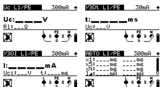
Рисунок 5.19: Тестирование УЗО
