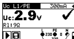
Рисунок 5.21: Пример результатов измерений контактного напряжения
