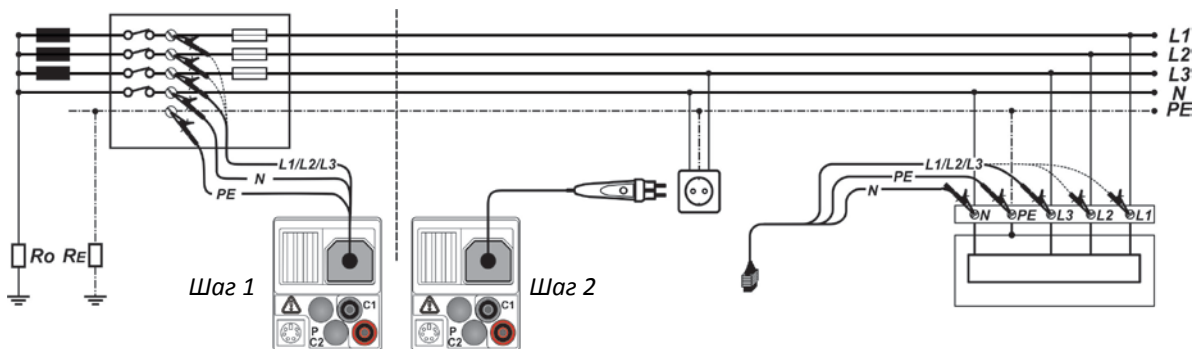
Рисунок 6.4: Настройка автоматической последовательности
