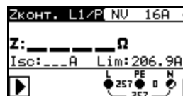
Рисунок 5.26: Импеданс короткозамкнутого контура
