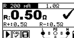
Рисунок 5.13: Пример результатов измерения R200 мА
