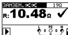
Рисунок 5.40: Пример результатов бесконтактного измерения сопротивления заземления
