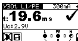
Рисунок 5.22: Пример результатов измерения времени отключения
