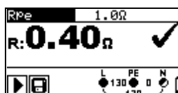
Рисунок 5.55: Пример результатов измерения сопротивления провода защитного заземления
