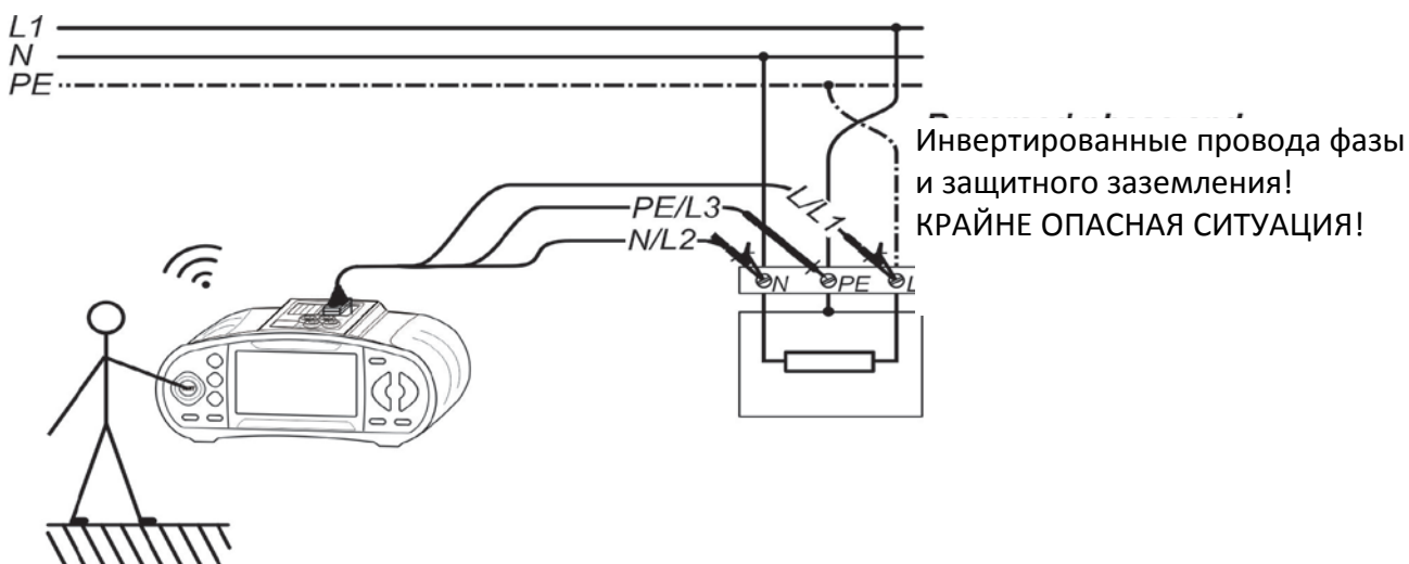
Рисунок 5.44: Инвертированные провода фазы и защитного заземления (L и PE) (применение 3-х проводного тестового кабеля)
