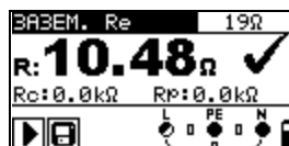
Рисунок 5.38: Пример результатов измерения сопротивления заземления
