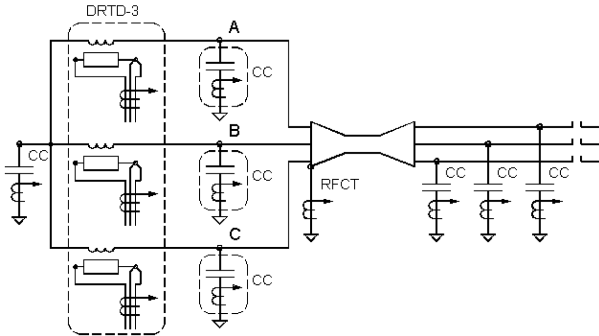
Рисунок 4 Возможные места установки ВЧ устройств контроля (комплектация MDR-M)
