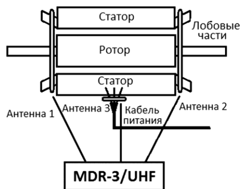
Рисунок 3 Схема расположения СВЧ-антенн (комплектация MDR-3/UHF)
