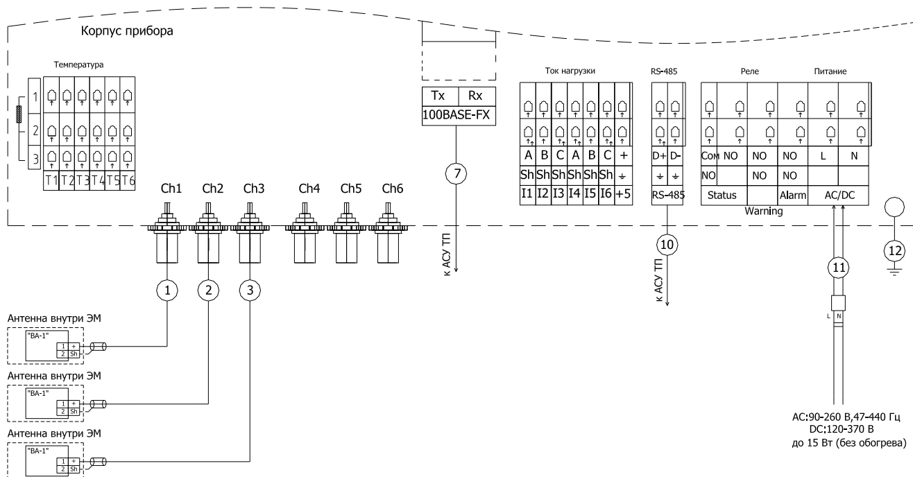
Рисунок 2 Пример типовой схемы подключений прибора в комплектации MDR-3/UHF
